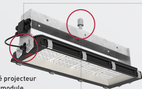
Unité projecteur à deux modules 100 000 lm – 120 000 lm
