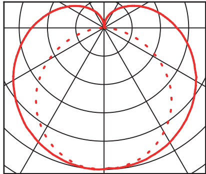
Apparecchio a plafone
